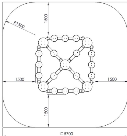
plattegrond
