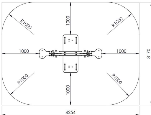
plattegrond
