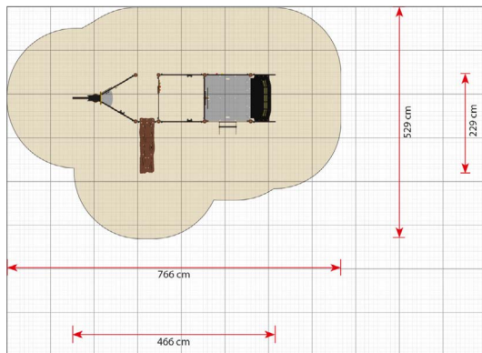
plattegrond
