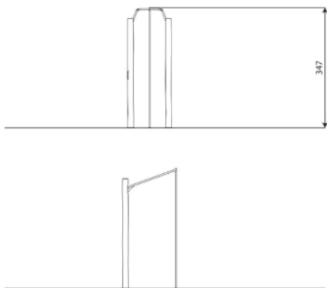
zijaanzicht
