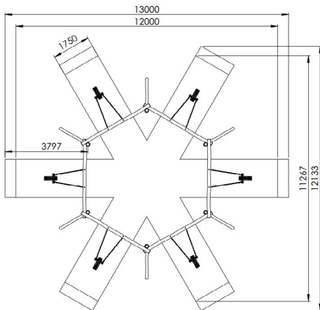
plattegrond
