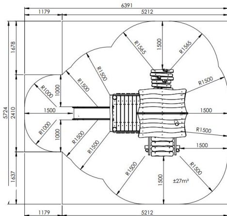
Plattegrond
