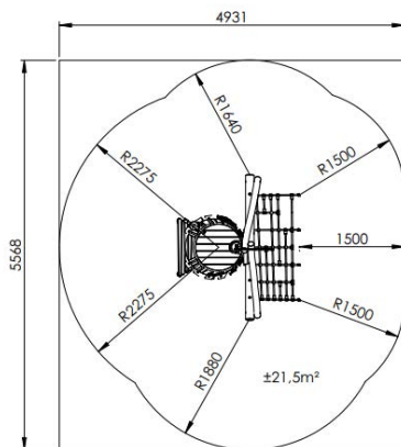
Plattegrond
