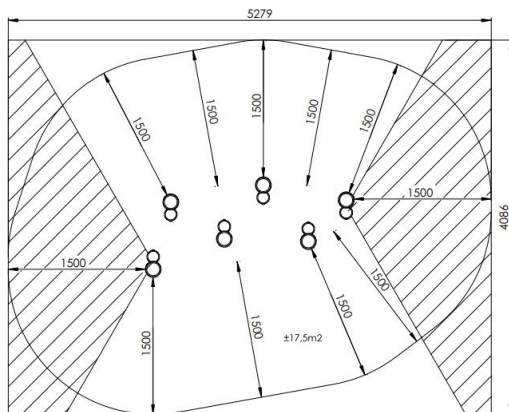
Plattegrond
