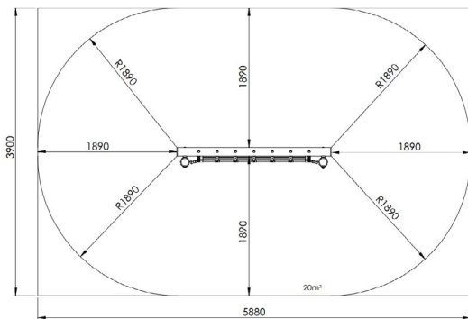
Plattegrond
