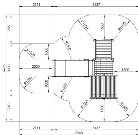
plattegrond
