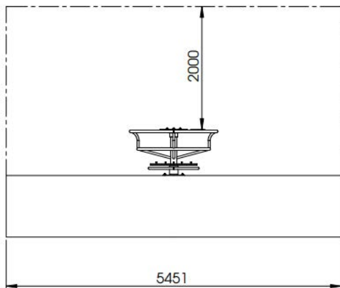
Zijaanzicht
