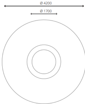
Plattegrond
