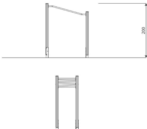
zijaanzicht
