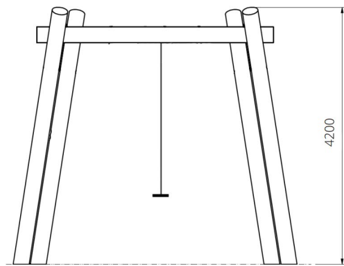
zijaanzicht
