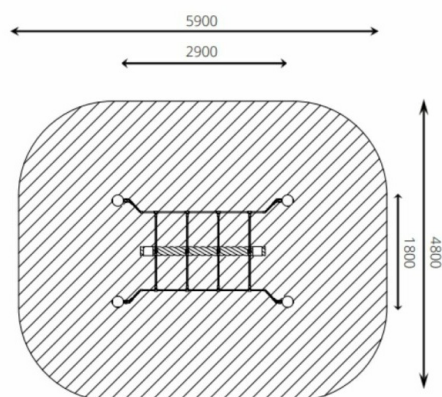
plattegrond
