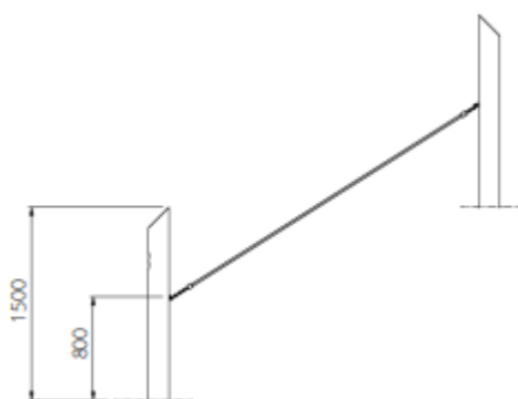
aanzicht
