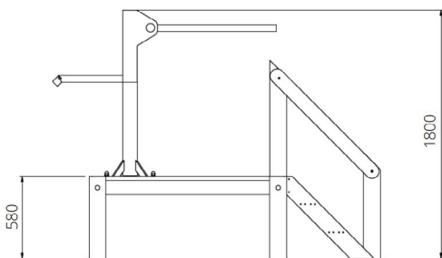
zijaanzicht
