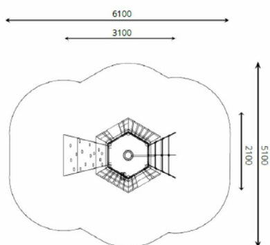
Plategrond
