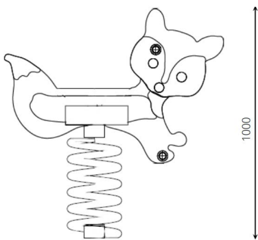
zijaanzicht
