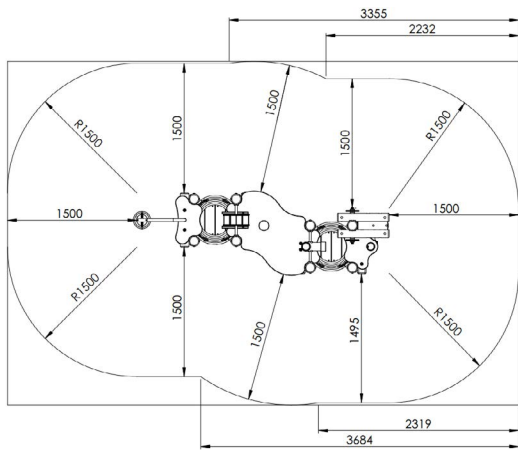
plattegrond
