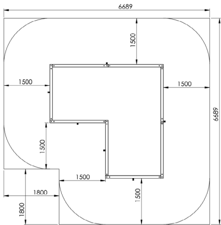
plattegrond
